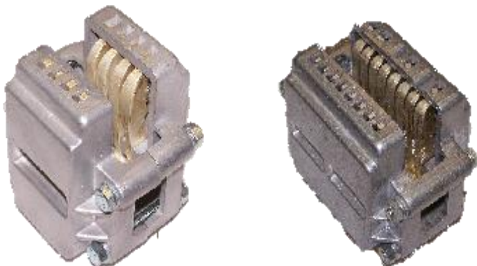
Flachkontakt für Bemessungsströme bis 630 A/ 1250 A
