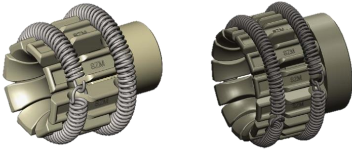
Tulpenkontakt für Bemessungsströme bis 1600 A/ 2500 A
